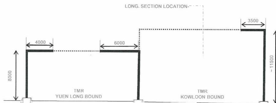
SECTION 14-14 SEMI-ENCLOSURE NM 21 (N.T.S.)
